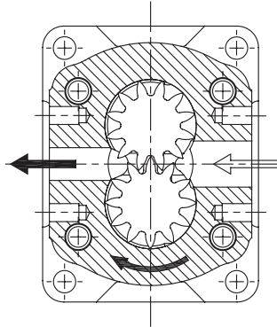
Sağ Dönüslü Pompa Clockwise Rotation
