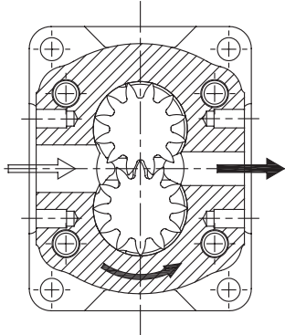
Sol Dönüslü Pompa Counter-clockwise Rotation
