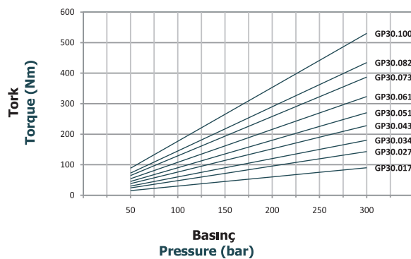
GP30 Pompaların Tork Eğrileri Torque Curves of GP30 Pumps
