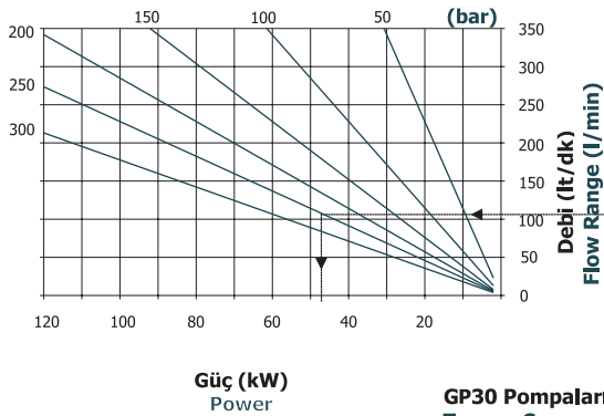
GP30 Pompaların Güç Eğrileri Power Curves of GP30 Pumps
