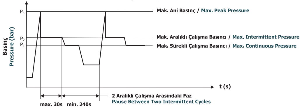
GP40 Pompaların Güç Eğrileri Power Curves of GP40 Pumps
