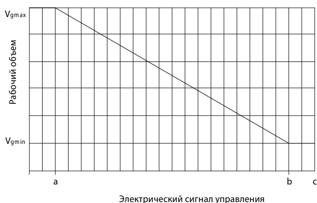
График регулирования 303...00D(00E)...
