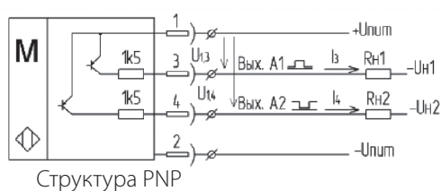
Рисунок 2 – Схема подключения нагрузки.
