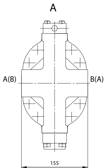
Расположение рабочих клапанов Опция 1:0 - 2 фланца по бокам по SAE
