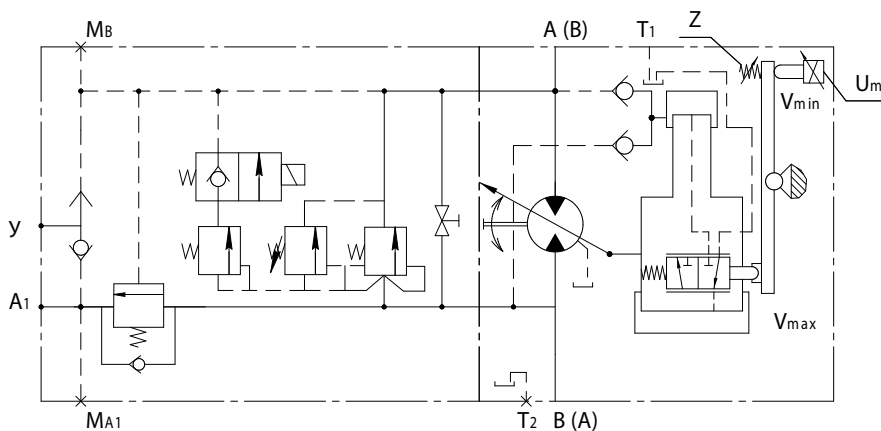
Гидравлическая схема мотора с пропорциональным негативным электроуправлением и пристыкованным блоком клапанов БК-03.20
