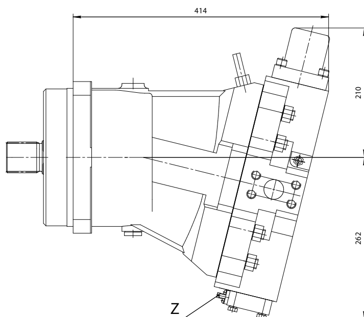
303.4.250.241 – гидромотор с регулятором по гиперболе с дополнительным негативным гидроуправлением
