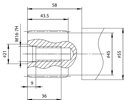
Опция G: 0 - шлицевое по ГОСТ 6033-80 50xh8x2x9g
