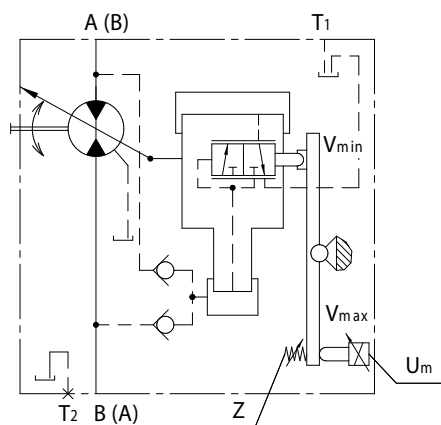
Гидравлическая схема 303...147...; 303...148...
