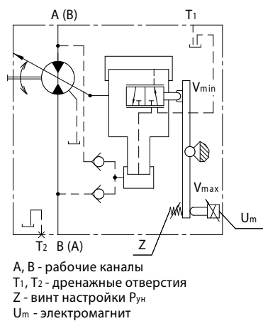
Гидравлическая схема 303...00F(00G)...
