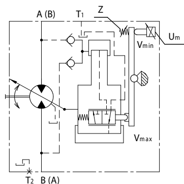
Гидравлическая схема 303...00D(00E)...
