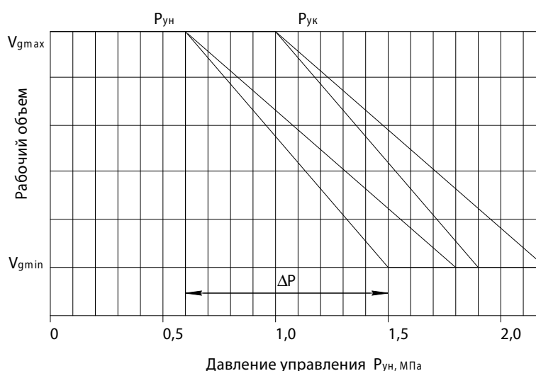
График регулирования 303...001...
