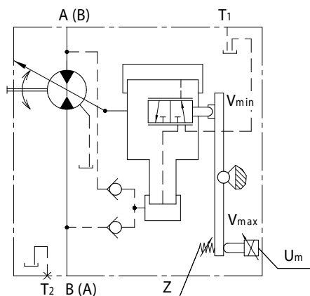
Гидравлическая схема 303...007(008)...
