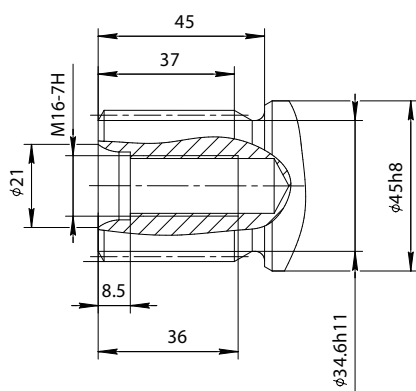
Опция G: 7 - шлицевое по DIN 5480 W40x2x30x18x9g
