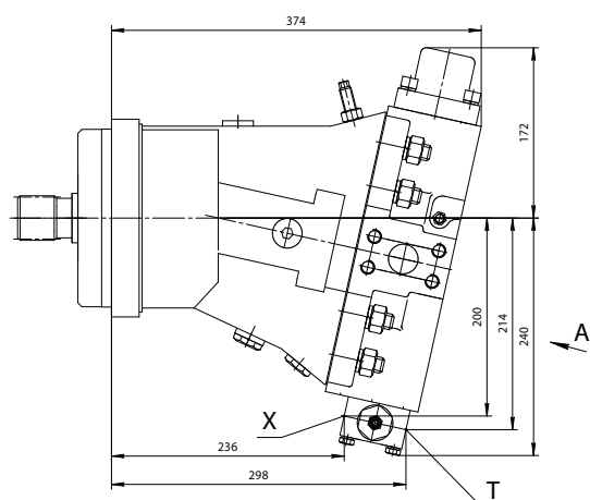
303.4.112.50D; 303.4.112.50E – гидромотор с пропорциональным негативным электроуправлением (12B, 24B)
