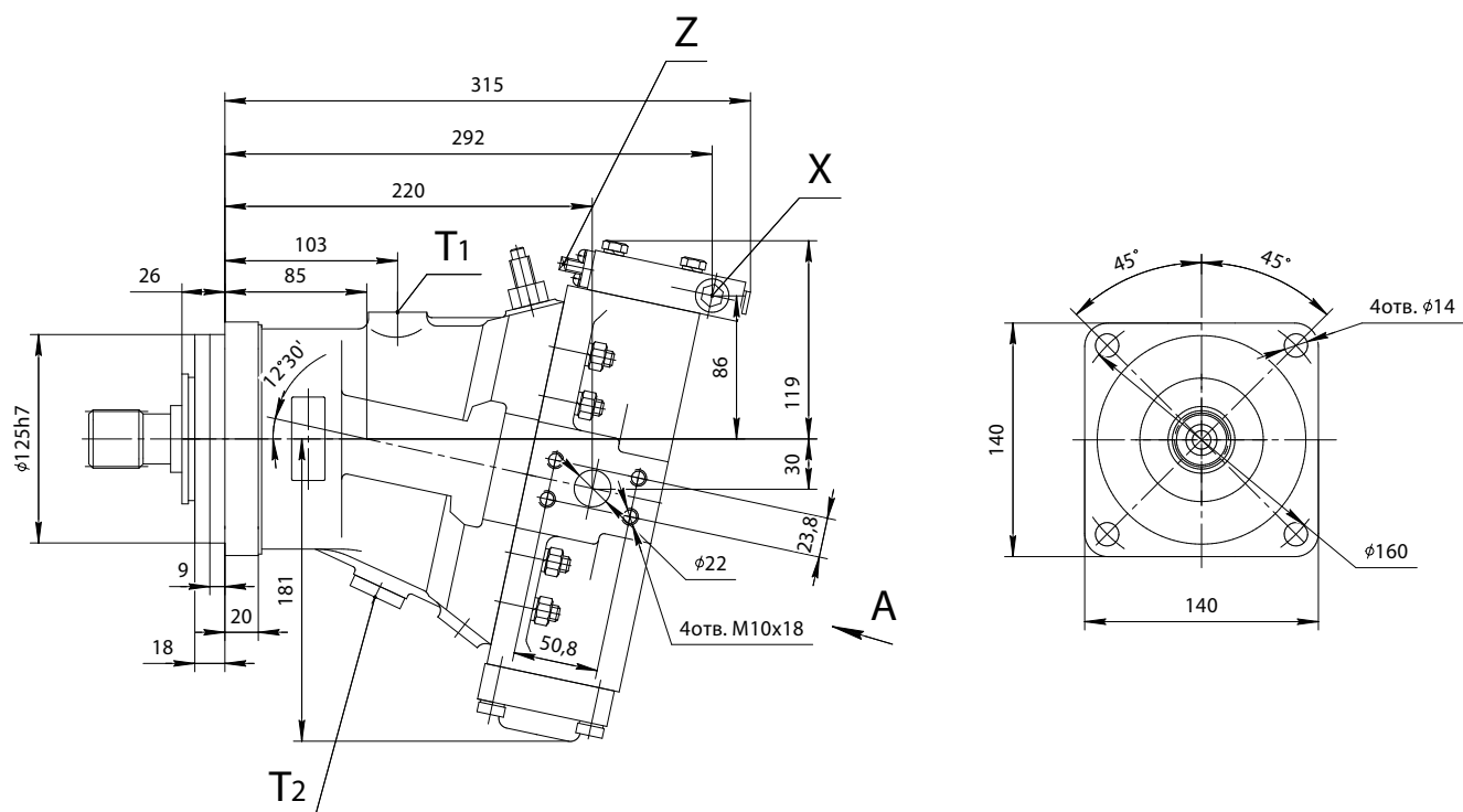
Расположение рабочих клапанов Опция 1:0 - 2 фланца по бокам по SAE
