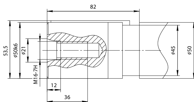
Опция G: 1 - шпоночное по DIN 6885 ϕ50k6 14x9x80
