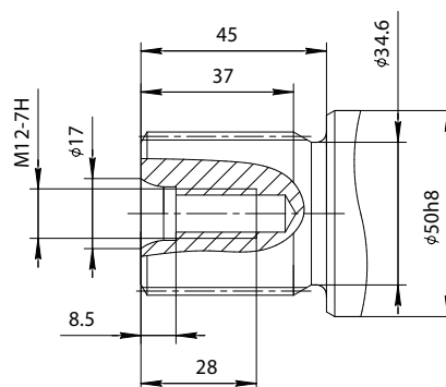
Опция G: 8 - шлицевое по DIN 5480 W40x2x30x18x9g
