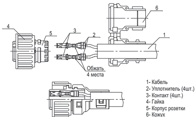
Рисунок 3 – Схема сборки и параметры соединителя.
