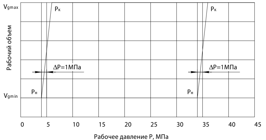
График регулирования 303...122...
