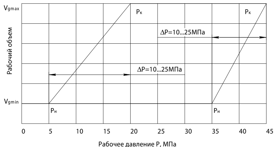
График регулирования 303...140...
