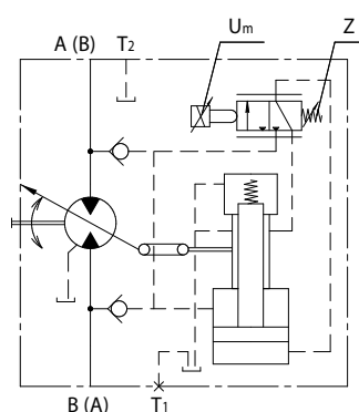
Гидравлическая схема 303...003(004)... для г/м с рабочим объемом 28 \text{см}^3/\text{об}
