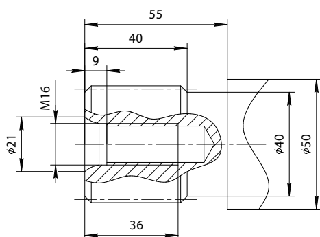
Опция G: 0 - шлицевое по ГОСТ 6033-80 45xh8x2x9g
