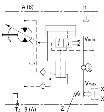
Гидравлическая схема 303...141...
