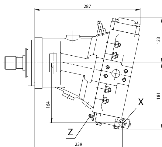
303.4.55.242 – гидромотор с регулятором по гиперболе с дополнительным позитивным гидроуправлением
