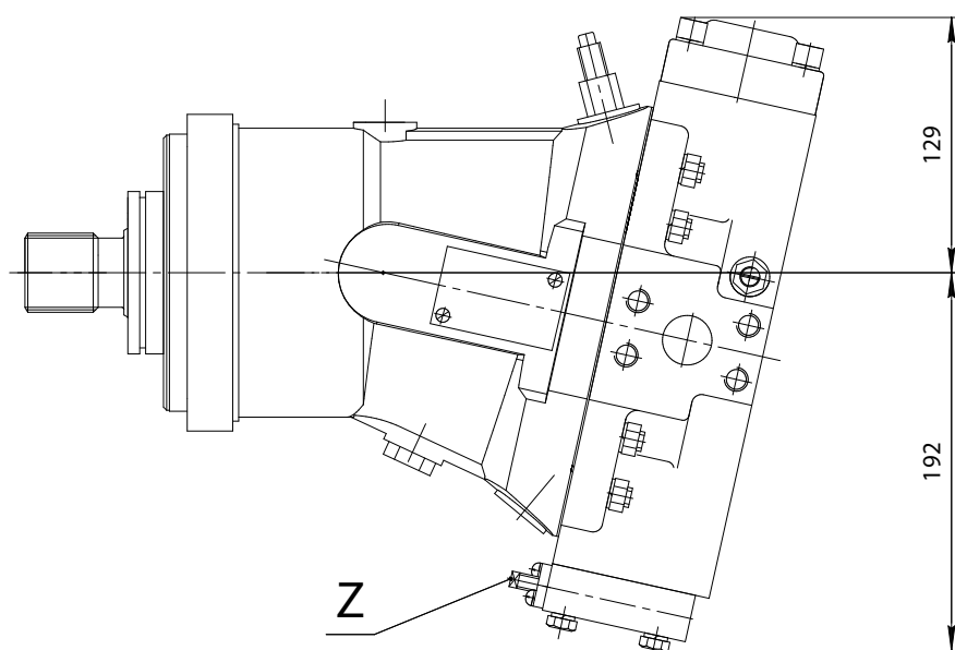
303.4.80.240 – гидромотор с регулятором по гиперболе
