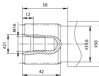
Опция G: 8 - шлицевое по DIN 5480 W45x2x30x21x9g
