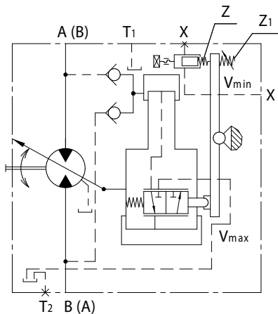
Гидравлическая схема 303...002...
