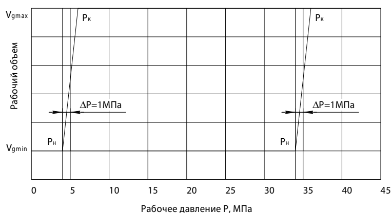
График регулирования 303...120...
