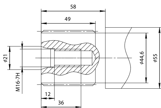
Опция G: 8 - шлицевое по DIN 5480 W50x2x30x24x9g
