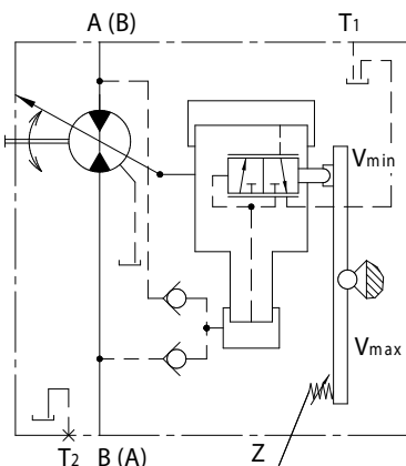
Гидравлическая схема 303...140...
