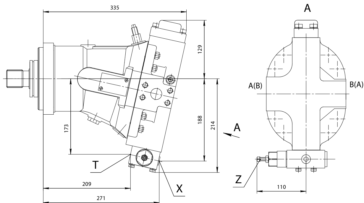
303.4.107.222 – гидромотор с регулятором постоянного давления с дополнительным пропорциональным позитивным гидроуправлением
