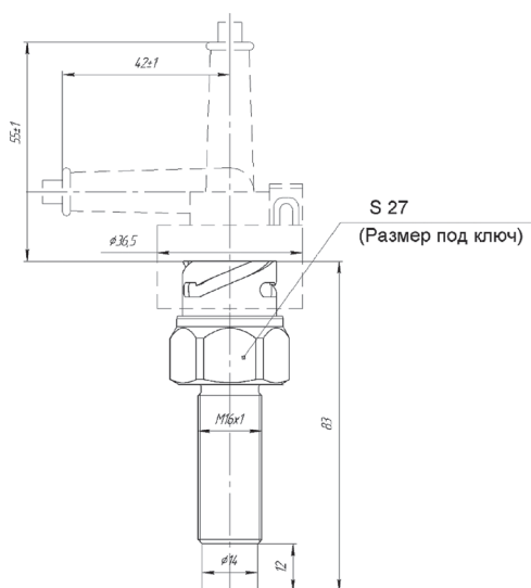
Рисунок 1 – Габариты датчика.
