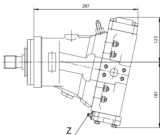
303.4.55.241 – гидромотор с регулятором по гиперболе с дополнительным негативным гидроуправлением
