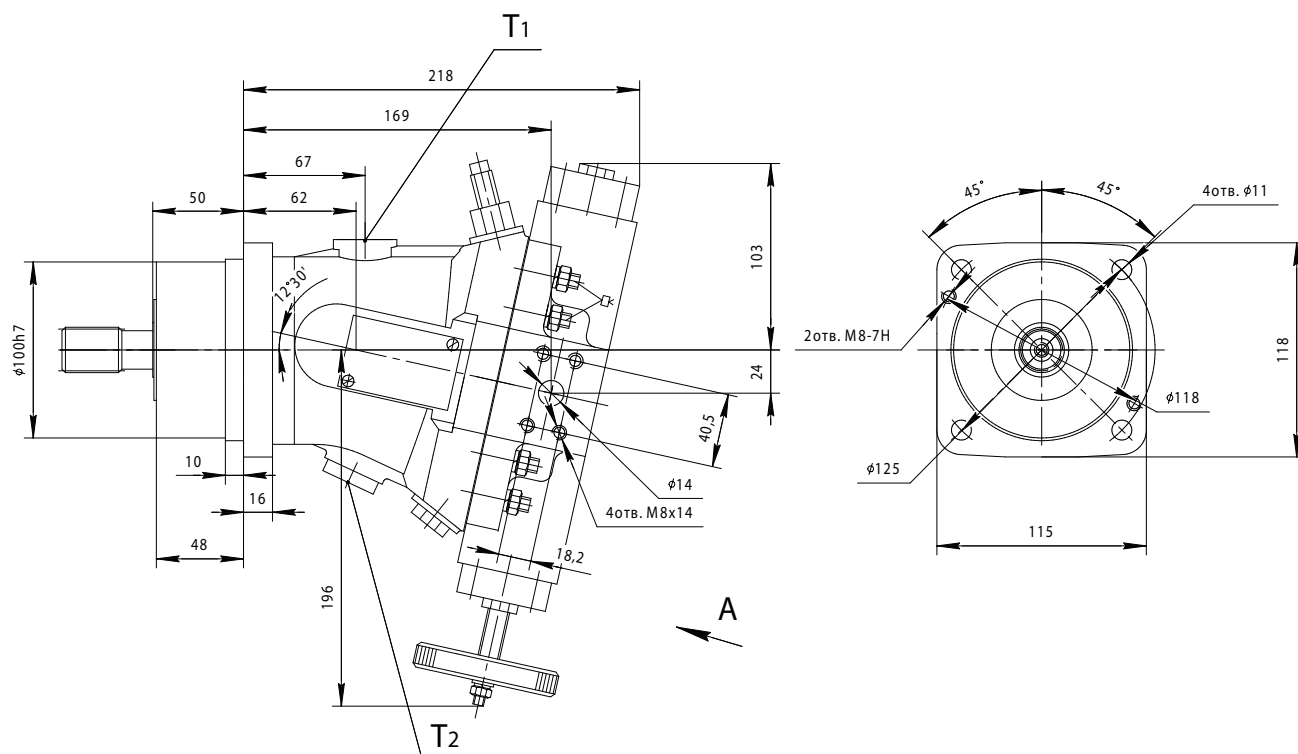
Расположение рабочих клапанов Опция 1:0 - 2 фланца по бокам по SAE
