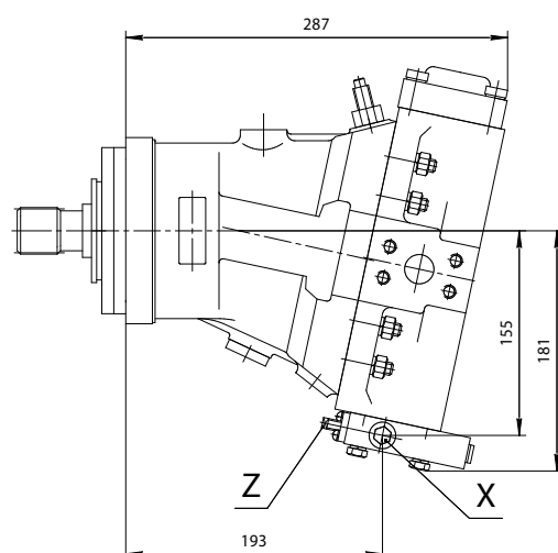
303.4.55.242 – гидромотор с регулятором по гиперболе с дополнительным позитивным гидроуправлением
