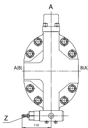
303.4.160.222 – гидромотор с регулятором постоянного давления с дополнительным позитивным гидроуправлением
