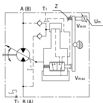
Гидравлическая схема 303...003(004)... для г/м с рабочим объемом 55, 56, 80, 107, 112, 160, 250 \text{см}^3/\text{об}
