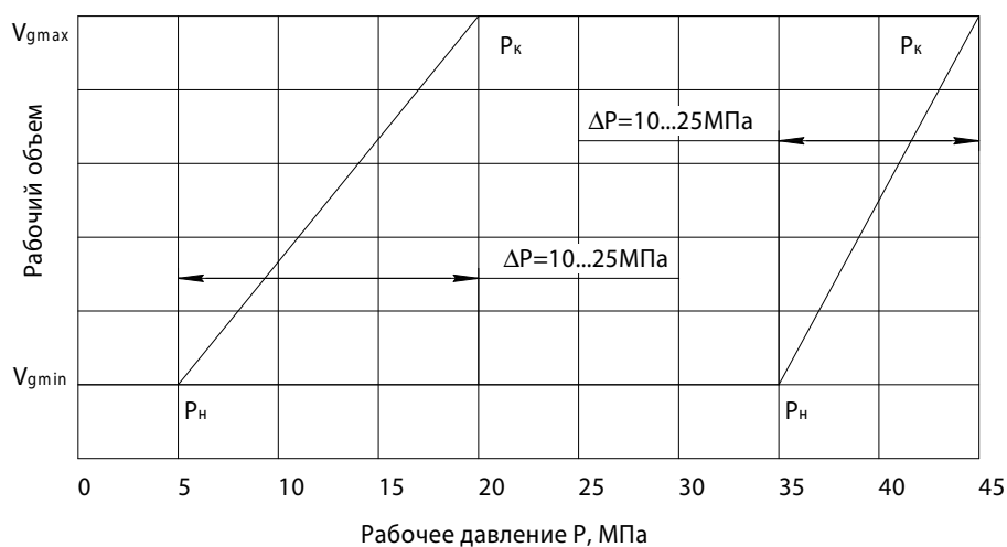
График регулирования 303...141...
