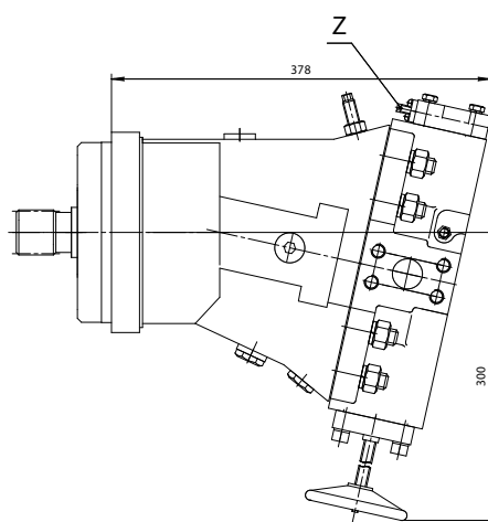
303.4.160.576 – гидромотор с механическим регулированием рабочего объема
