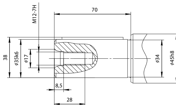
Опция G: 1 - шпоночное по DIN 6885 \phi 35k6 10x8x56
