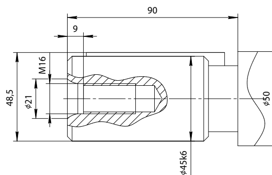
Опция G: 1 - шпоночное по DIN 6885 φ45k6 14x9x70
