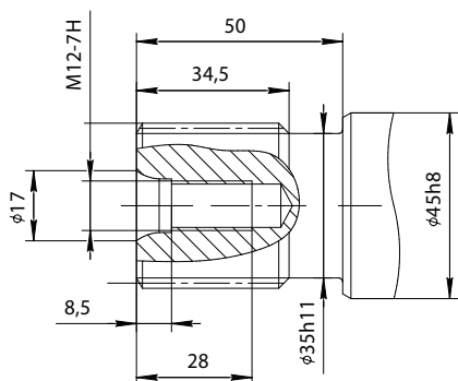
Опция G: 0 - шлицевое по ГОСТ 6033-80 40xf7x2x9g
