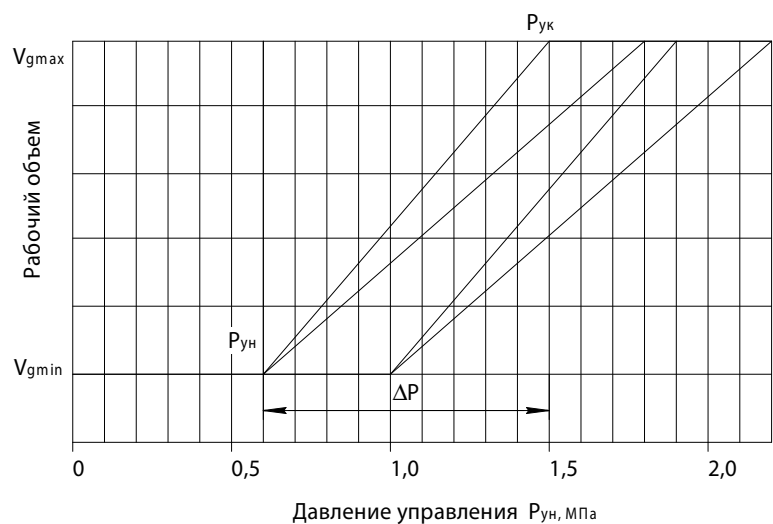
График регулирования 303...002...
