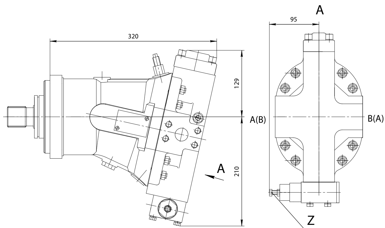
303.4.80.220 – гидромотор с регулятором постоянного давления
