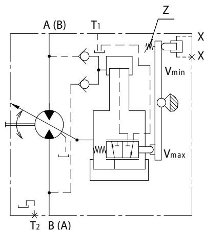
Гидравлическая схема 303...001...
