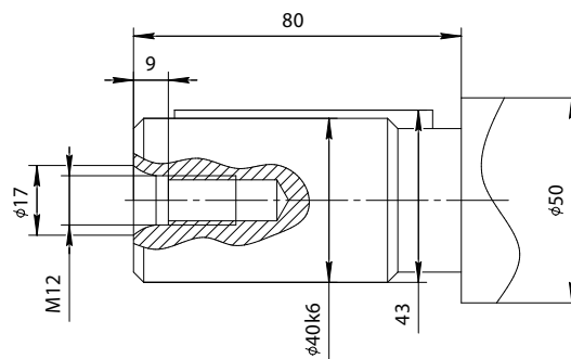
Опция G: 1 - шпоночное по DIN 6885 φ40k6 12x8x63
