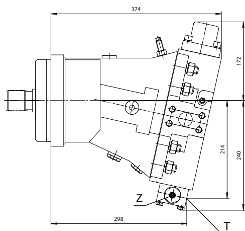
303.4.160.222 – гидромотор с регулятором постоянного давления с дополнительным позитивным гидроуправлением
