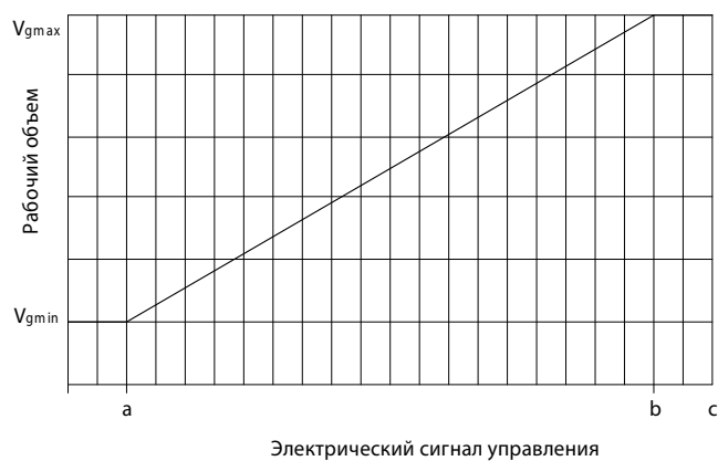
График регулирования 303...00F(00G)...
