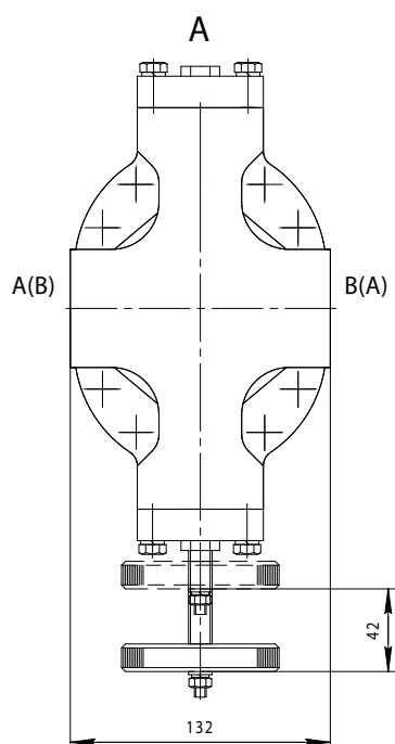
Расположение рабочих клапанов Опция 1:0 - 2 фланца по бокам по SAE
