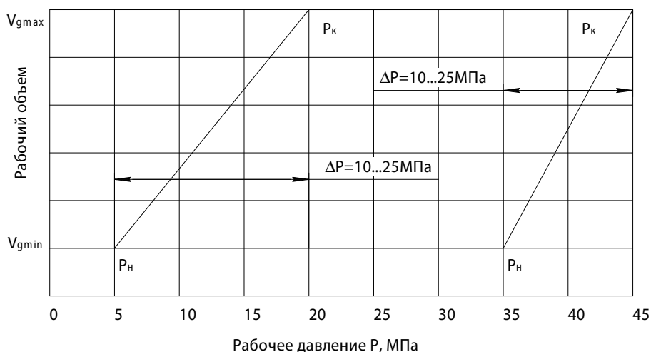
График регулирования 303...147...; 303...148...
