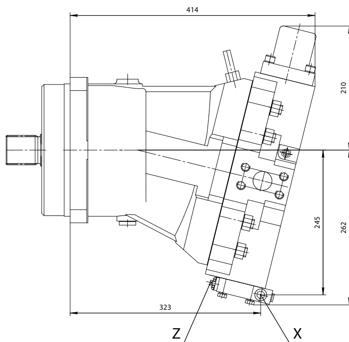
303.4.250.241 – гидромотор с регулятором по гиперболе с дополнительным негативным гидроуправлением
