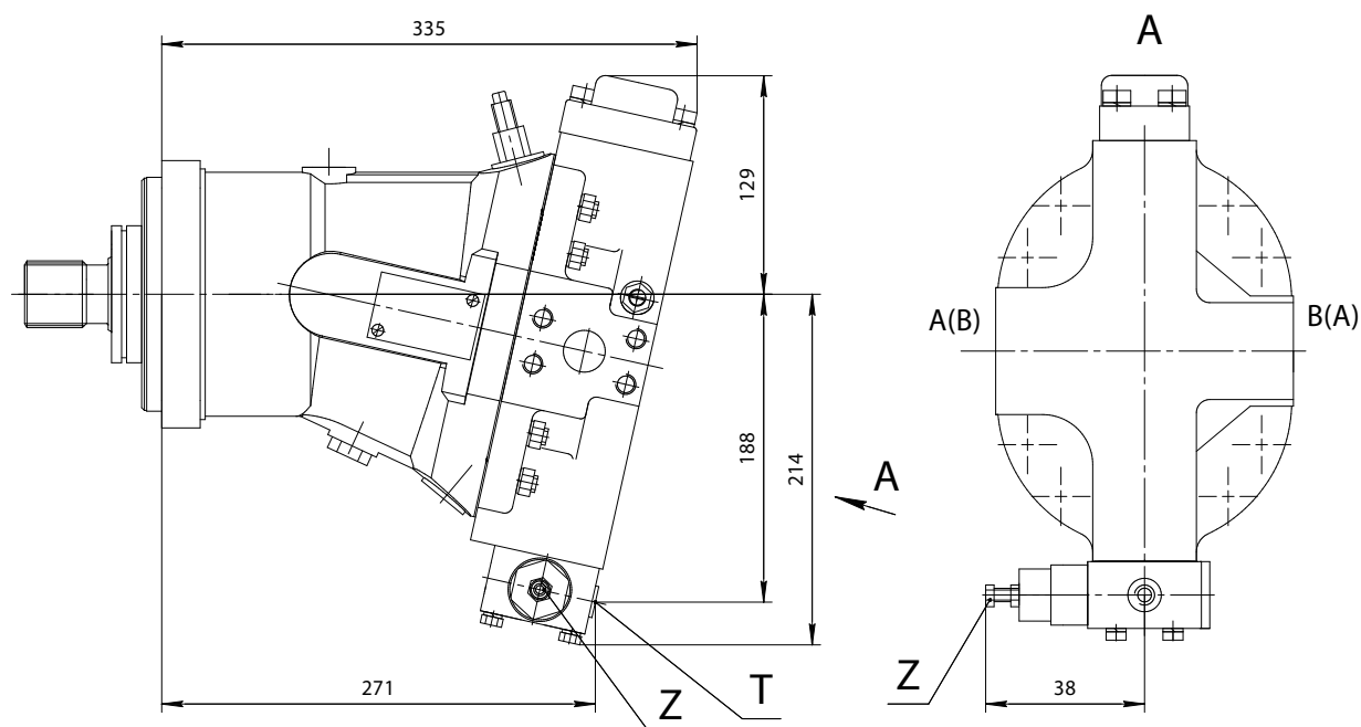
303.4.107.220 – гидромотор с регулятором постоянного давления
